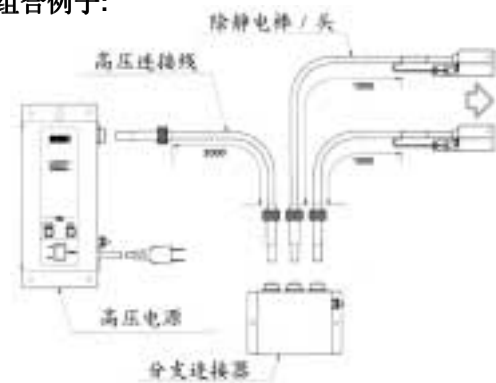
BOS 型: 除静电棒 轻便实用, 便于安装和拆卸 一般用途, 印刷机, 纺织机, 包装机及各类塑料机 (棒 41x45.5mm)
